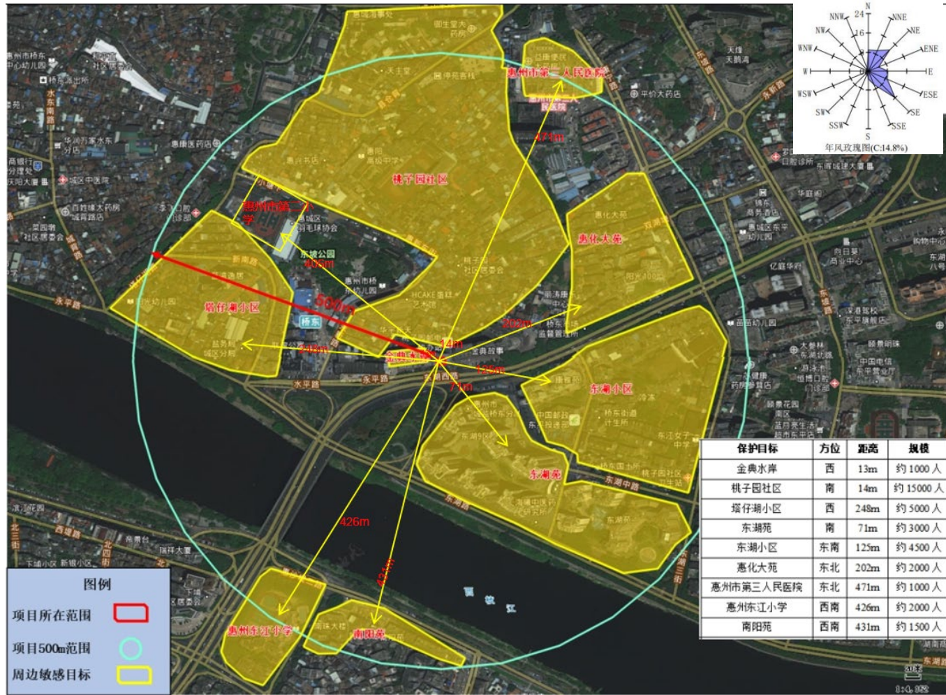
附图 3 项目周边 500m 评价范围示意图
