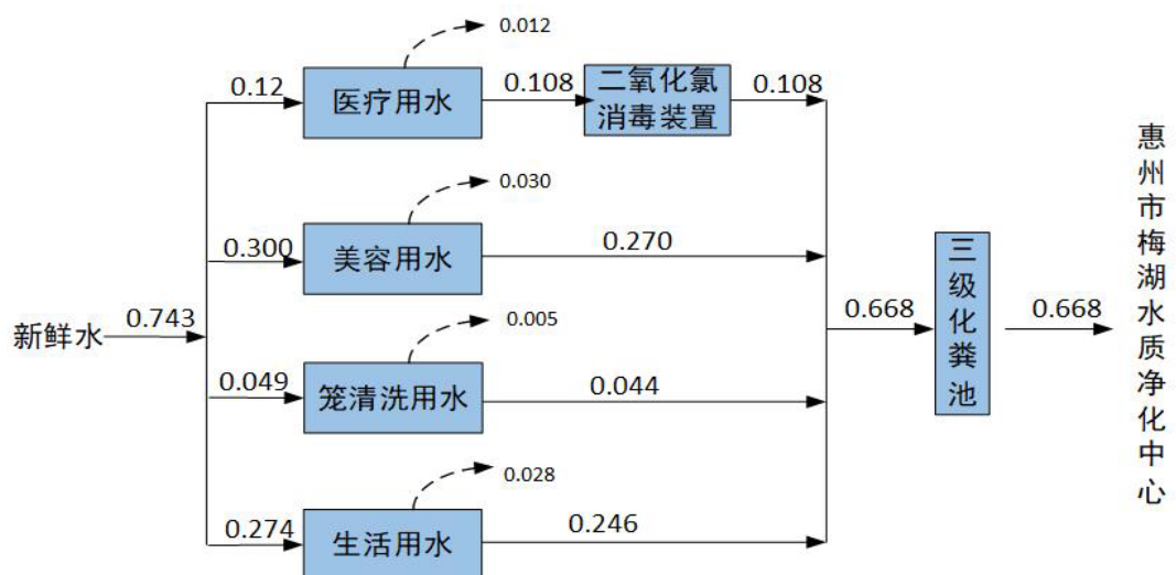
图 2-1 项目运营期水平衡图 ( \text{m}^3/\text{d} )
